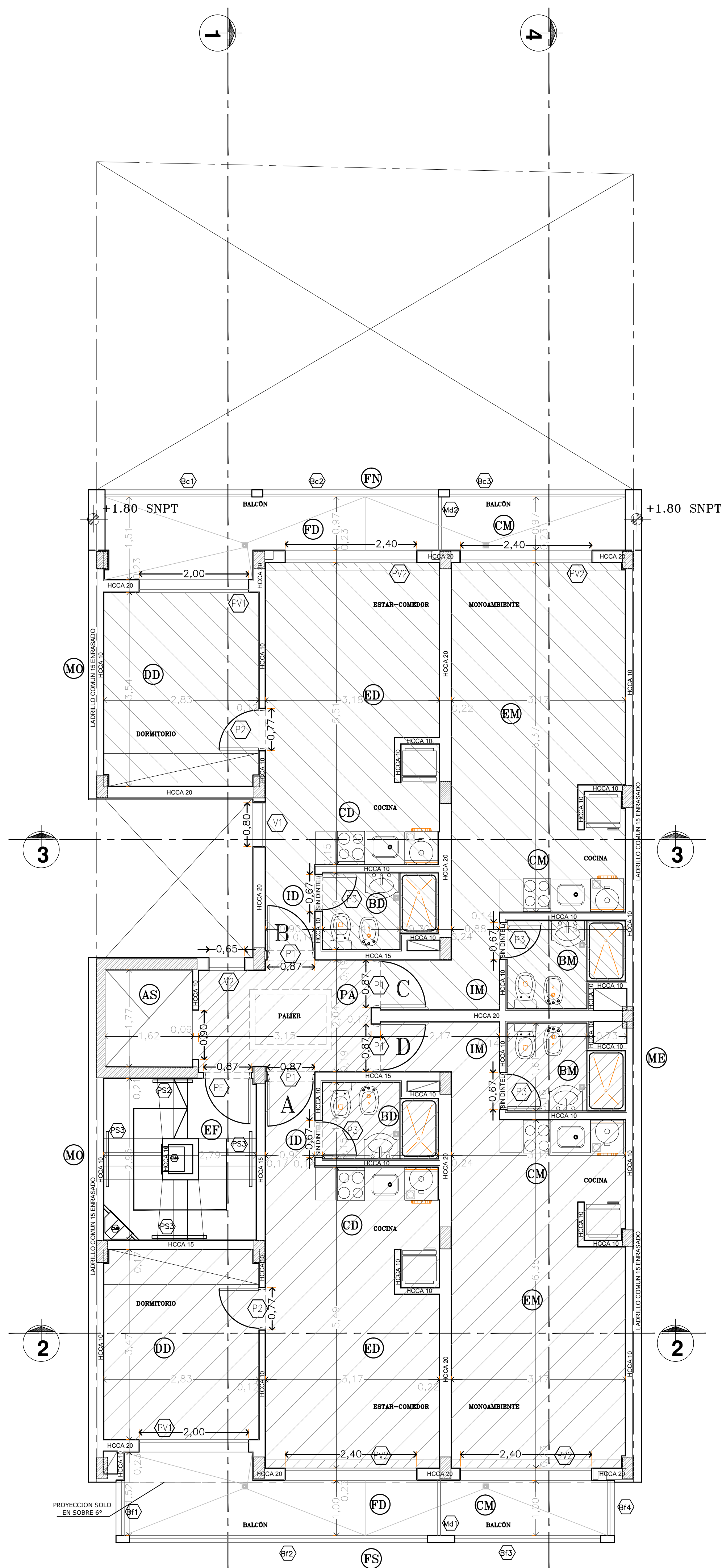
PLANTA TIPO (2° A 6°)
